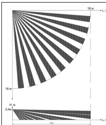
Рис. 3. Вид зоны обнаружения извещателя
