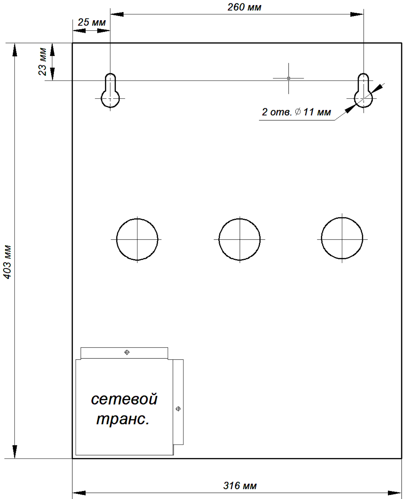
Рисунок 2 – Установочный чертеж ППК «А16-512» (корпус выпускается начиная с 2012 года)
