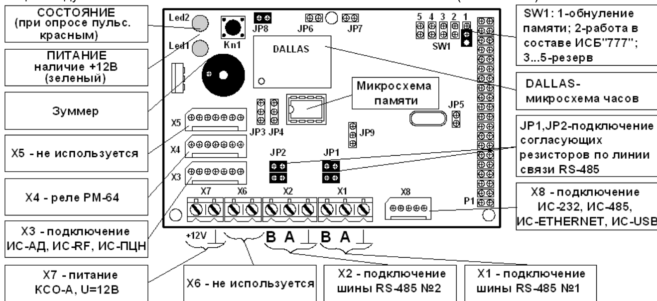
Рисунок 15 - Внешний вид модуля процессорного КСО-А
