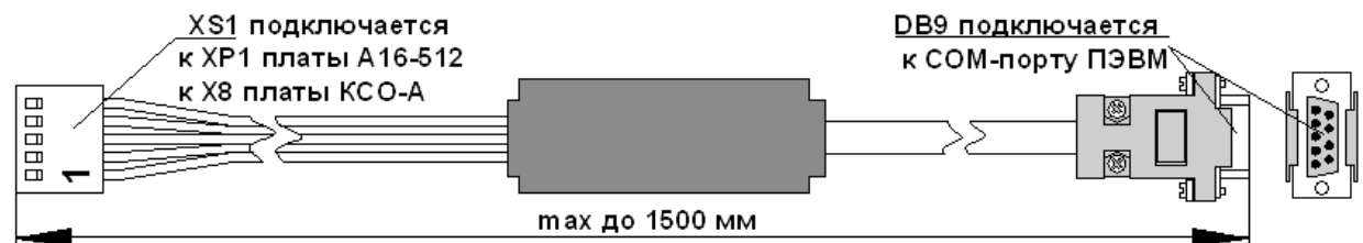
Рисунок 28 – Внешний вид модуля согласования ИС-232
