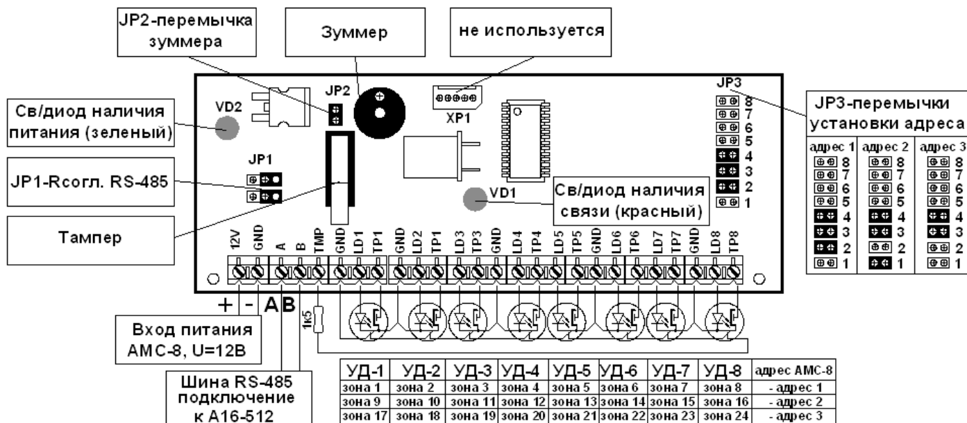
Рисунок 13 - Внешний вид модуля устройств доступа АМС-8
