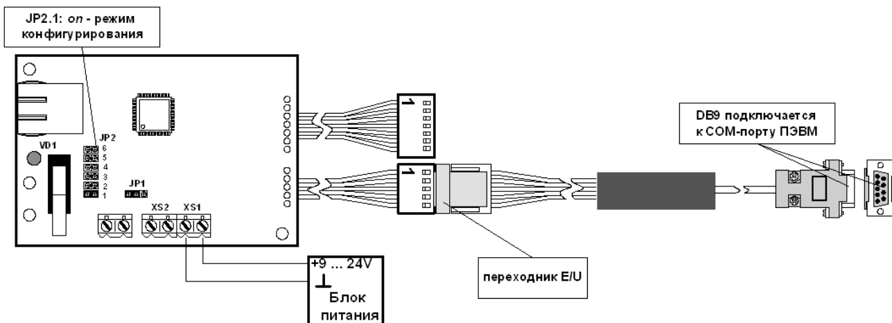
Рисунок 35 – Подключение модулей IC-ETH/485 и IC-232
