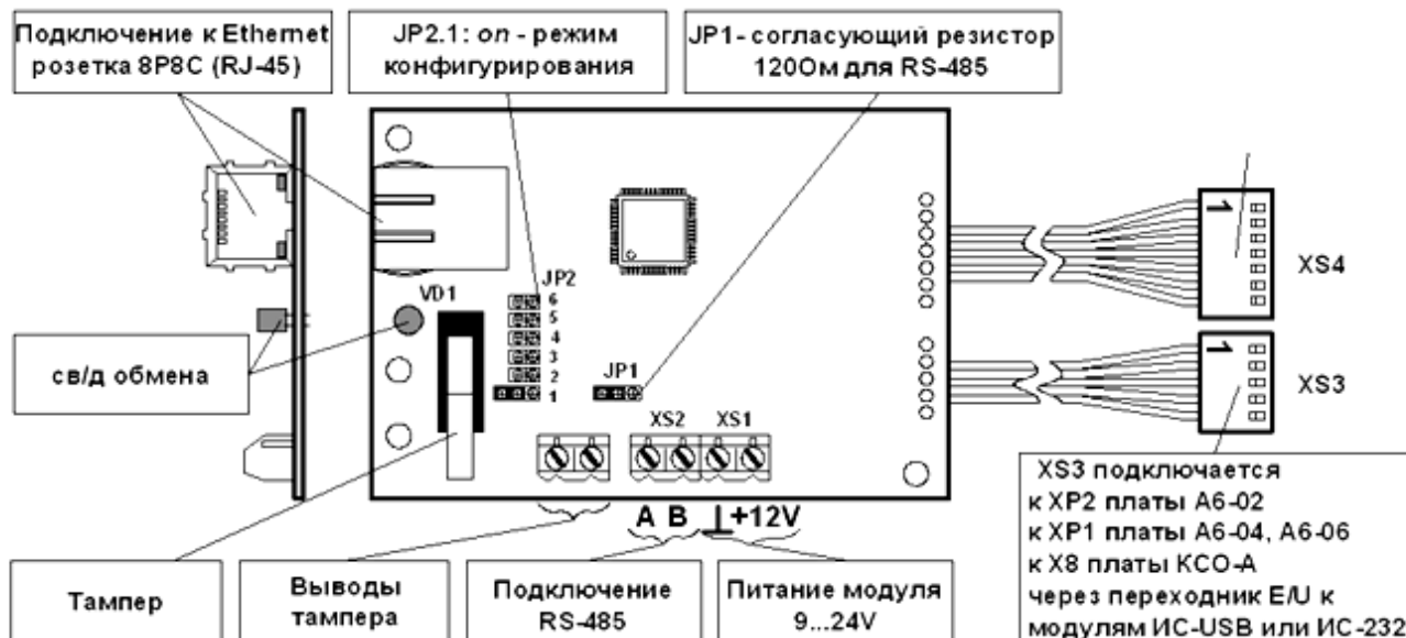
Рисунок 32 – Внешний вид модуля ИС-ETH/485.
