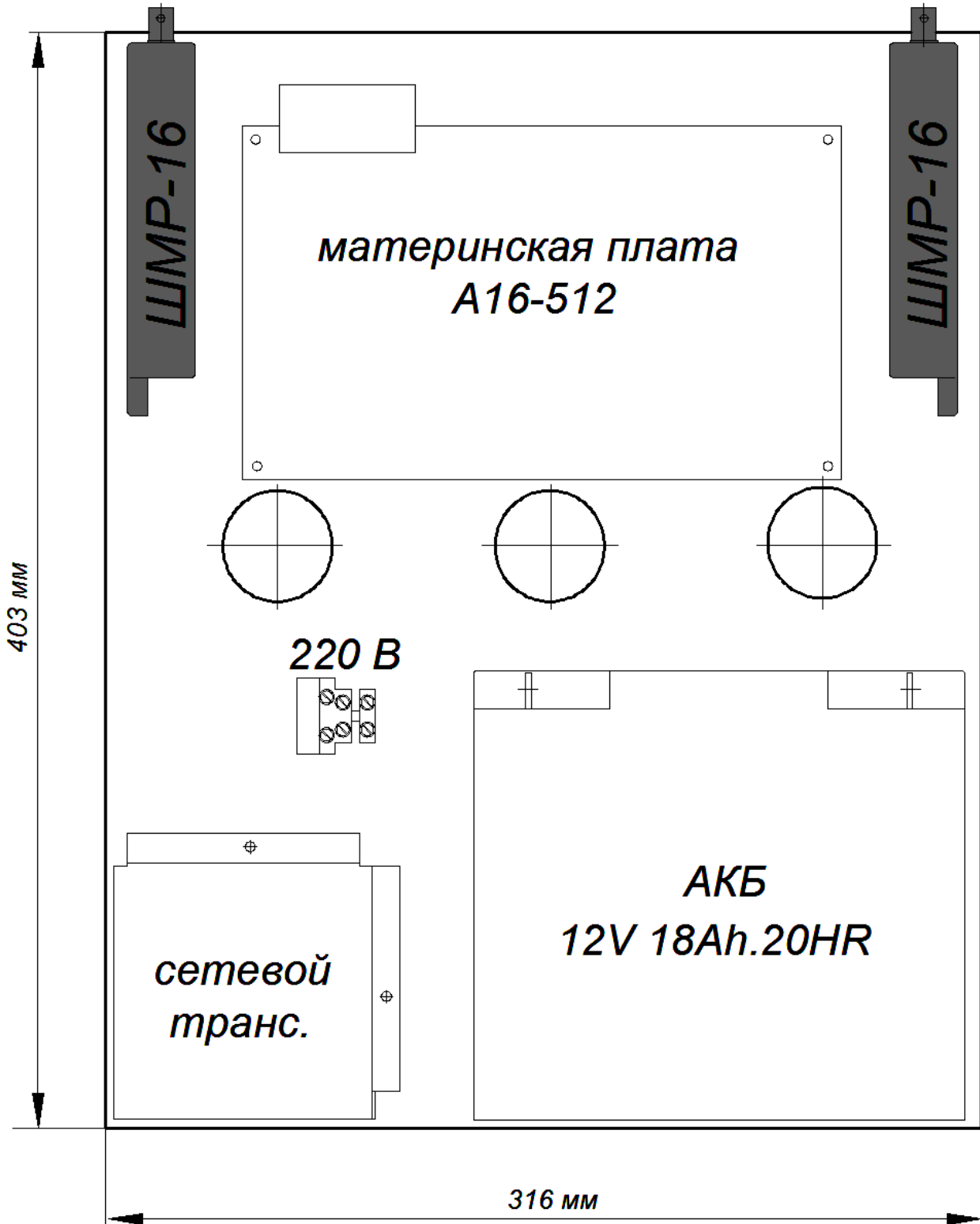
Рисунок 3 – Варианты установки коммуникатора ШМР-16 (корпус выпускается начиная с 2012 года)
