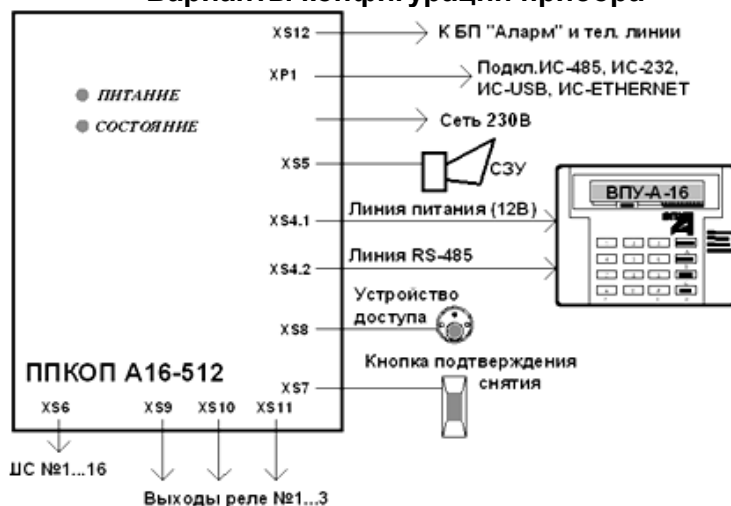
Рисунок 1 - Конфигурация прибора «А16-512» в минимальной комплектации
