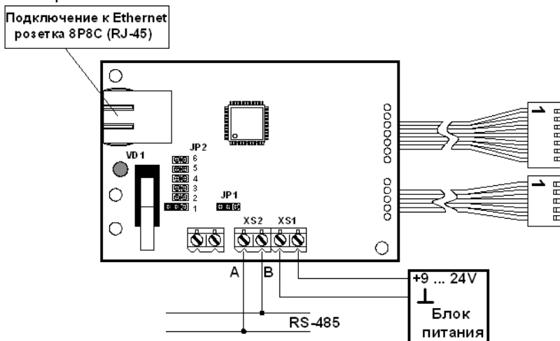
Рисунок 33 – Подключение модуля ИС-ETH/485 к RS-485.
