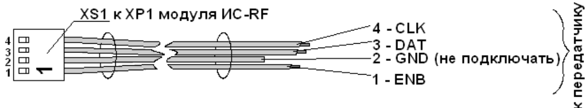
Рисунок 4 – Внешний вид шлейфа-адаптера при работе ППК «А16-512» в составе РСПИ «Андромеда» («PIMA»)
