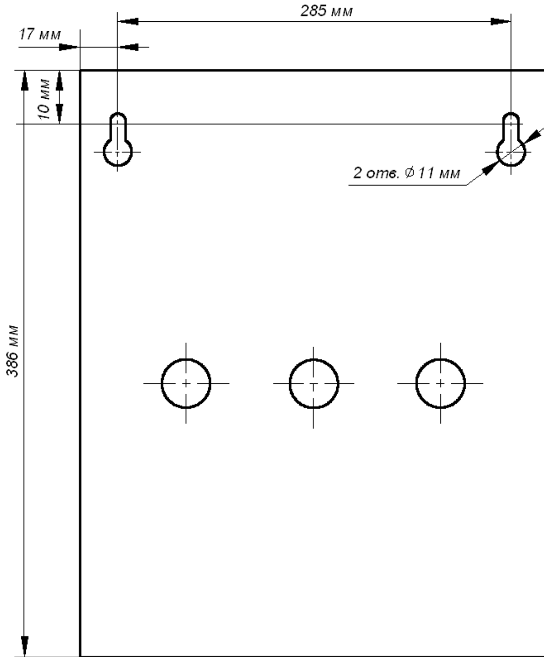
Рисунок 1 – Установочный чертеж ППК «А16-512» (корпус выпускался до 2012 года)
