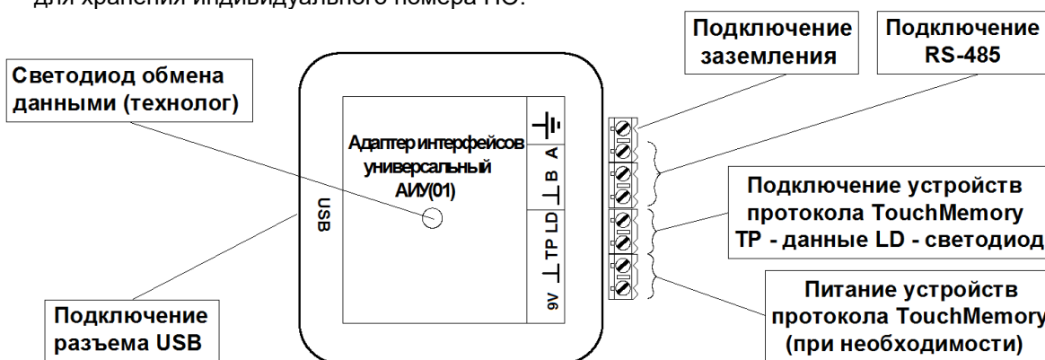
Рисунок 36 – Подключение модулей IC-ETH/485 и IC-232
