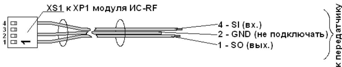
Рисунок 3 – Внешний вид шлейфа-адаптера при работе ППК «А16-512» в составе РСПИ «LARS» (KP Electronic Systems)
