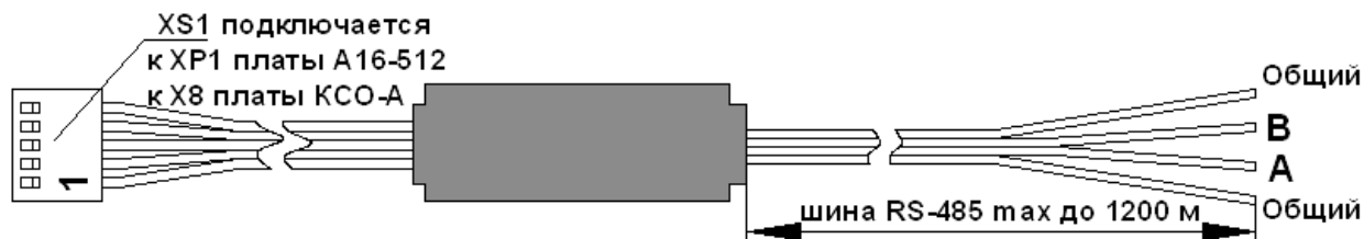
Рисунок 27 – Внешний вид модуля согласования ИС-485
