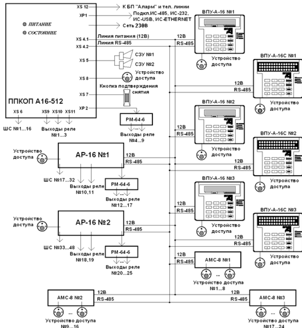
Рисунок 5 - Конфигурация ППК «А16-512» в максимальной комплектации
