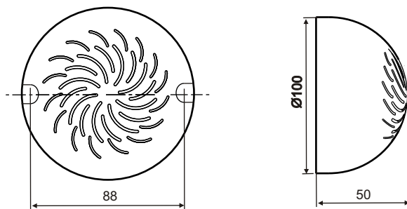
Рис.1. Габаритные и установочные размеры
