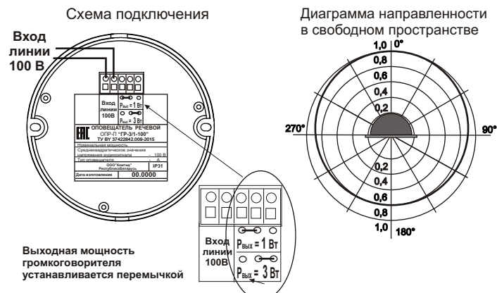
Рис.2 Схема подключения и диаграмма направленности оповещателя .
