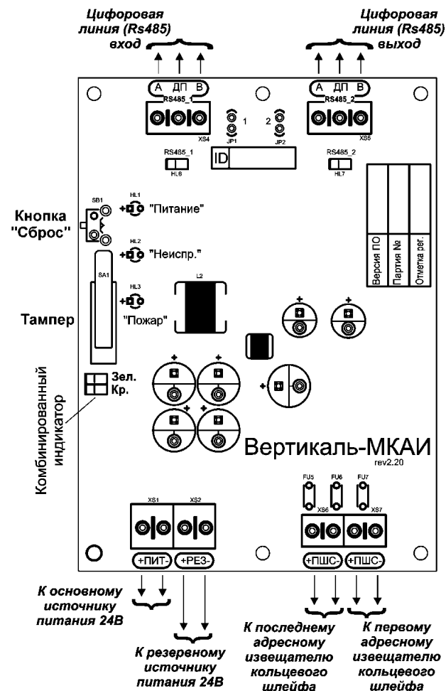
Рисунок 3 - Монтажная схема МКАИ
