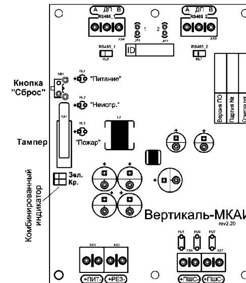
Рисунок 2 - Расположение индикаторов и кнопок на плате МКАИ
