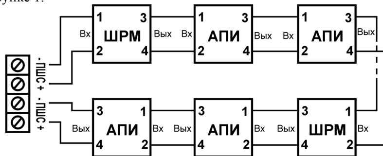
Рисунок 1- Схема включения извещателей в шлейф пожарной сигнализации
