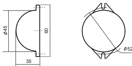
Рис.1. Габаритные и установочные размеры оповещателя
