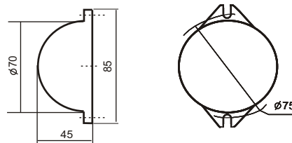
Рис.1. Габаритные и установочные размеры оповещателя
