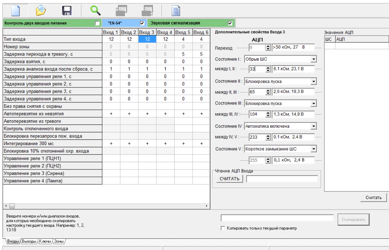
Рисунок 6. Вход «автоматика»
