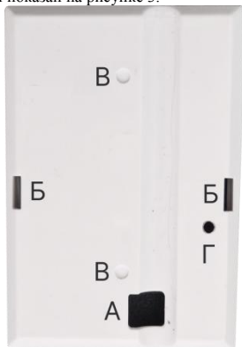
Рис. 3. Внешний вид основания корпуса
