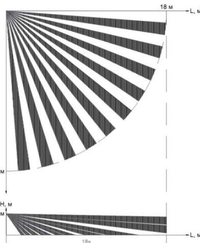
Рис. 3 Вид зоны обнаружения извещателя по ИК-каналу
