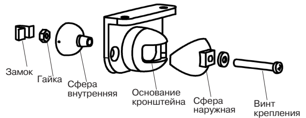
Рисунок 3 – Детали кронштейна
