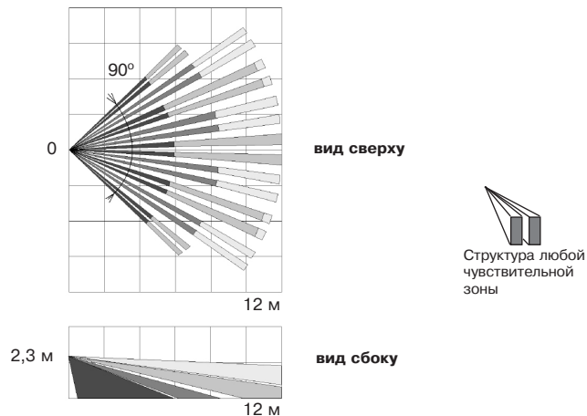
Рисунок 1 – Диаграмма зоны обнаружения извещателя
