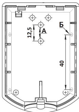
Рисунок 3 – Расположение монтажных отверстий на основании извещателя
