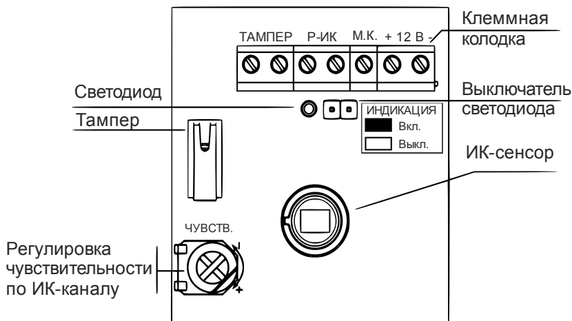
Рисунок 2 - Внешний вид платы извещателя
