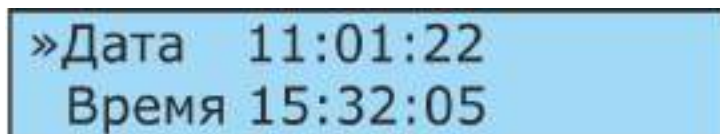
Рисунок 70. Подменю «дата/время»
