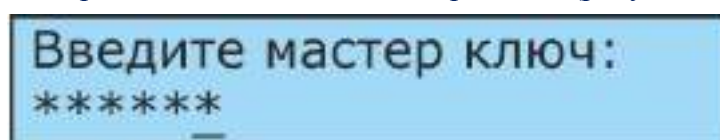
Рисунок 24.Ввод мастер-кода
