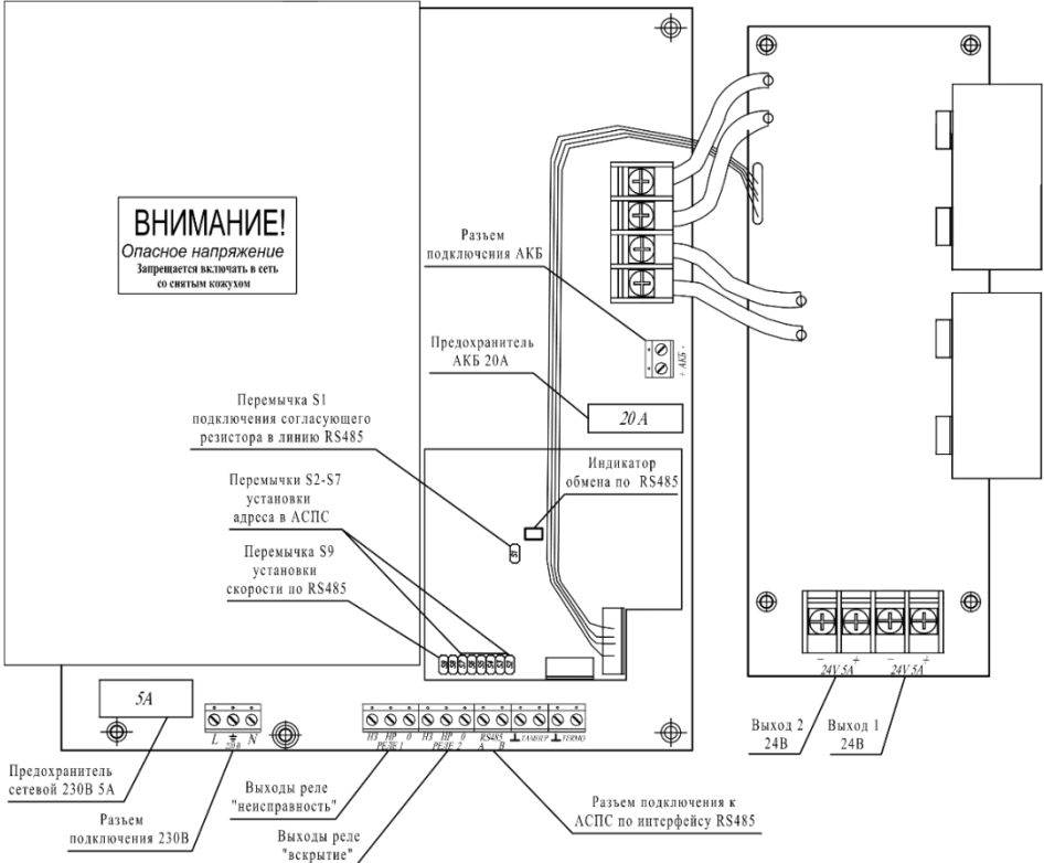
Рис. 1. Расположение контактных колодок, предохранителей, установочных элементов БП
