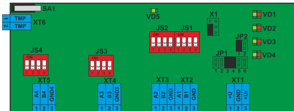
Рис. 2 Внешний вид платы Р485
