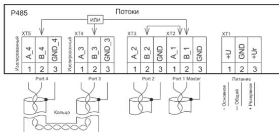
Рис.3. Режим работы «Петля (кольцо)»
