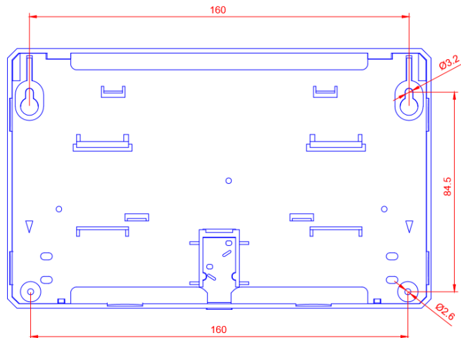
Рис.11 Установочный эскиз основания корпуса Р485
