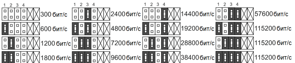
Рис.7 Установка скорости передаваемой информации
