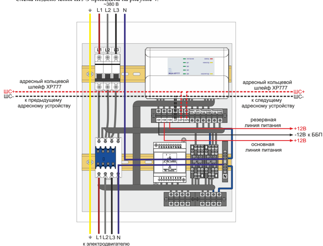
Рис. 4 Схема подключения ШУЭ
