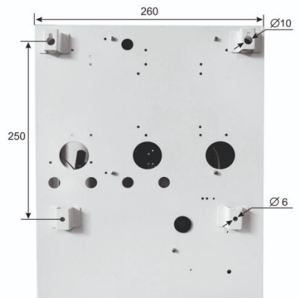
Рис.2 Установочные размеры
