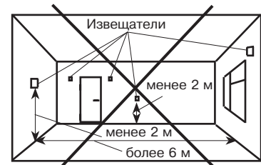
Рисунок 7 – Нерекомендуемые места установки извещателя
