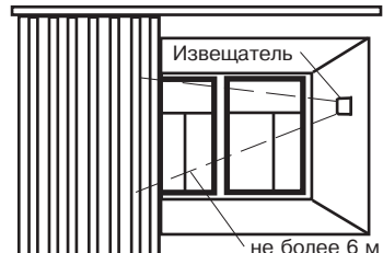
Рисунок 6 – Установка извещателя между стеклом и занавесями (жалюзи)
