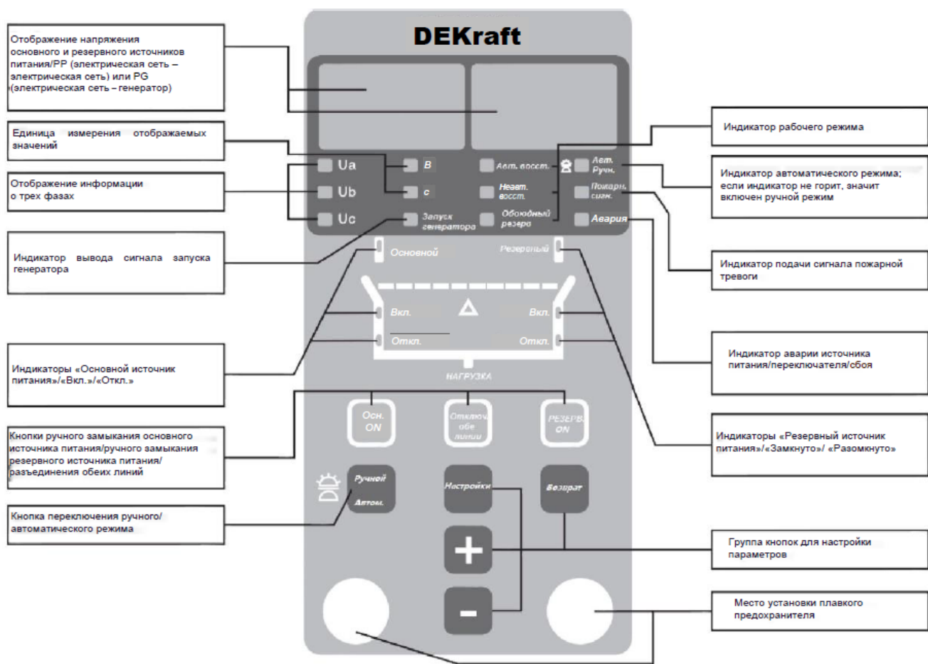
Рисунок 2. Лицевая панель контроллера блока.
