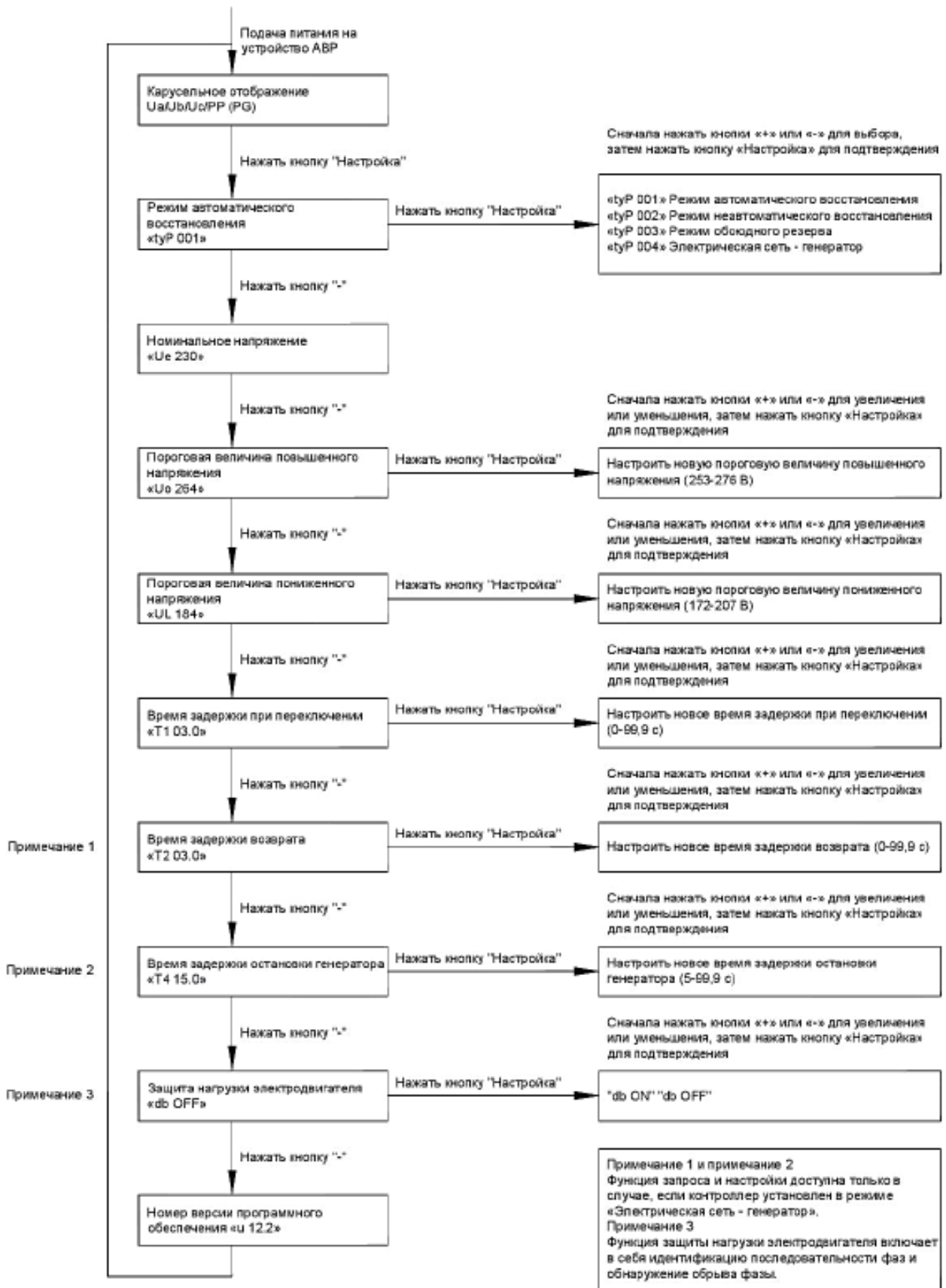
Рисунок 4. Процесс настройки контроллера блока.
