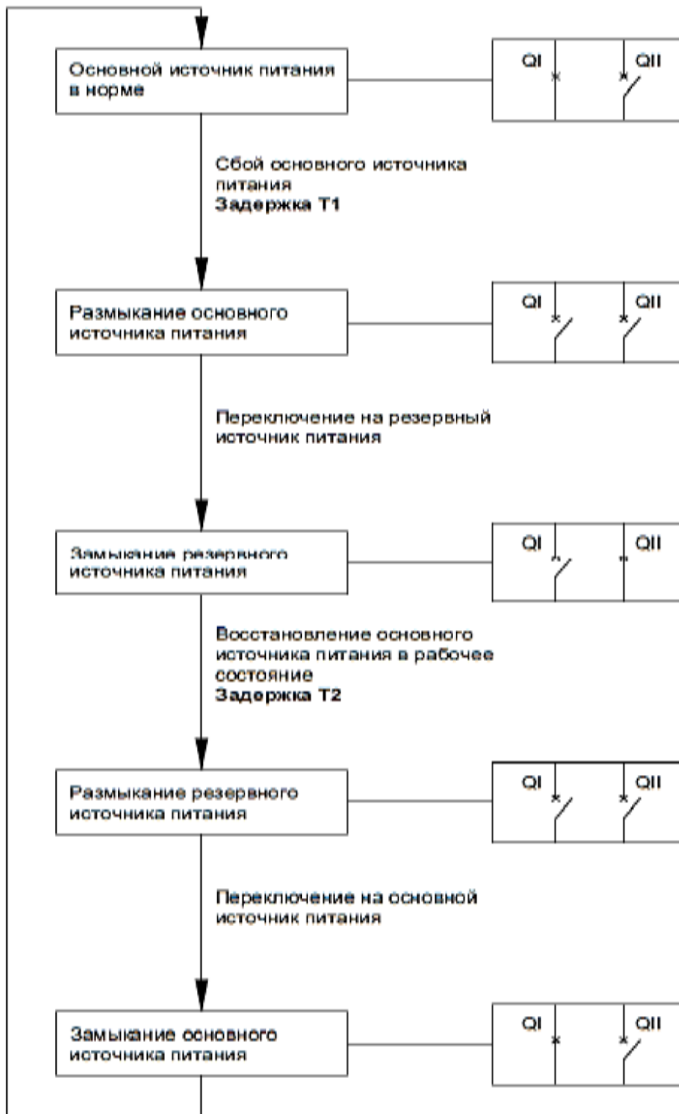
Рисунок 1. Описание работы алгоритма блока.
