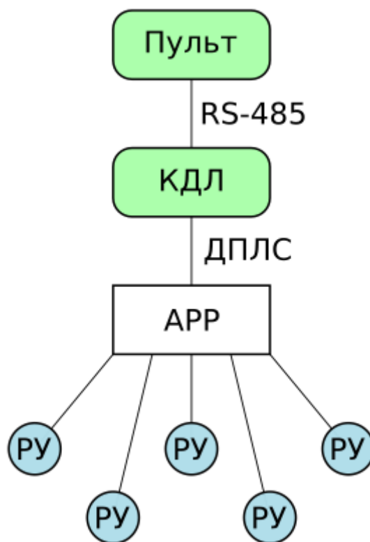
Рисунок 1.1 Блок-схема подключения адресных радиоканальных устройств
