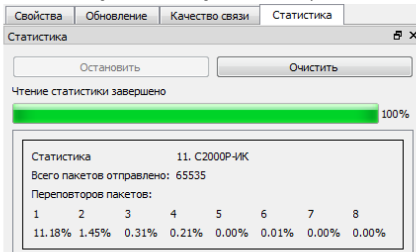
Рисунок 2.16 Статистика радиообмена
