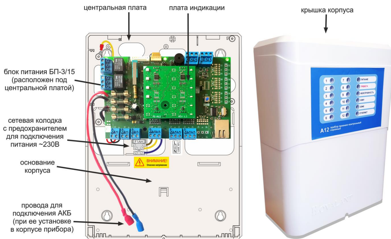
Рис. 1. Внешний вид и состав ППКО
