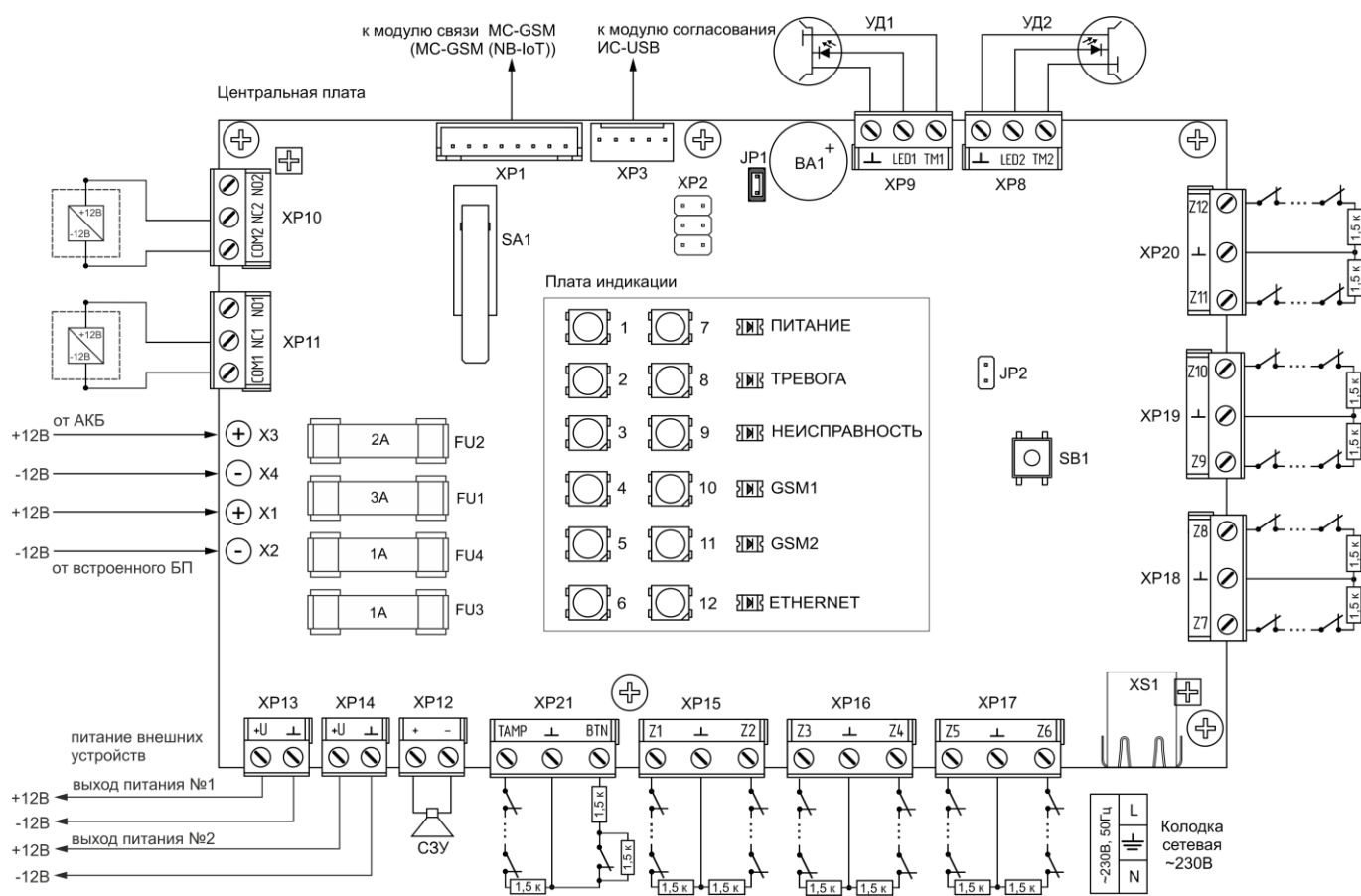
Рис. 2. Схема подключения ППКО А12/12
