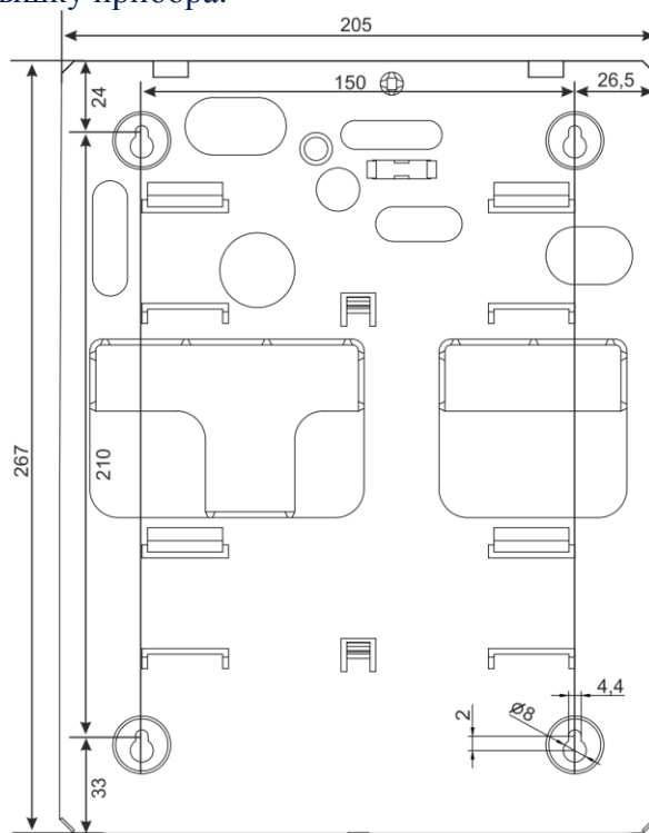
Рис. 5. Установочный чертеж основания корпуса ППКО серии «A12»
