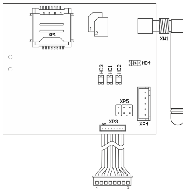
Рис. 3. Внешний вид модуля связи МС-GSM
