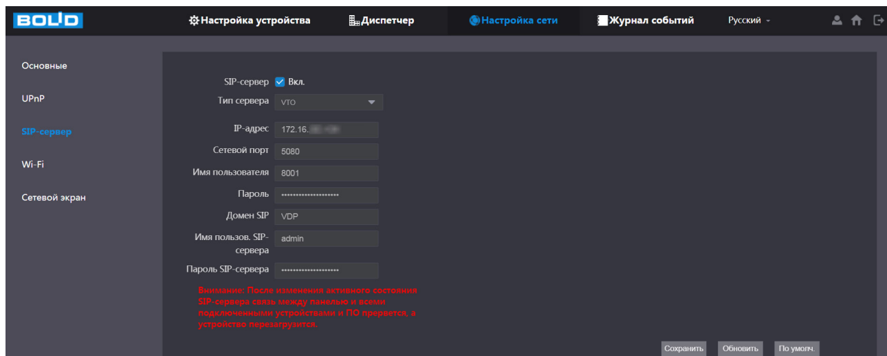
Рисунок 10.12 – Настройка SIP-сервера
