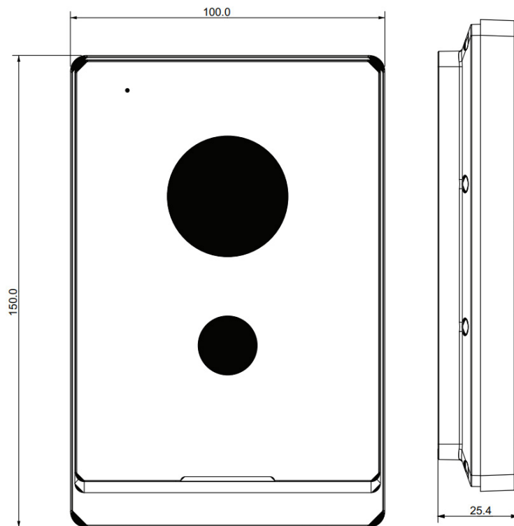
Рисунок 4.1 – Габаритные размеры
