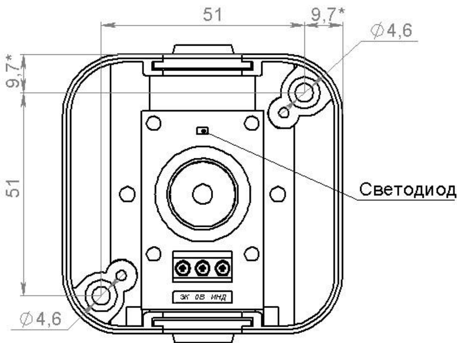
Рис. 3 Установочные размеры считывателя.
