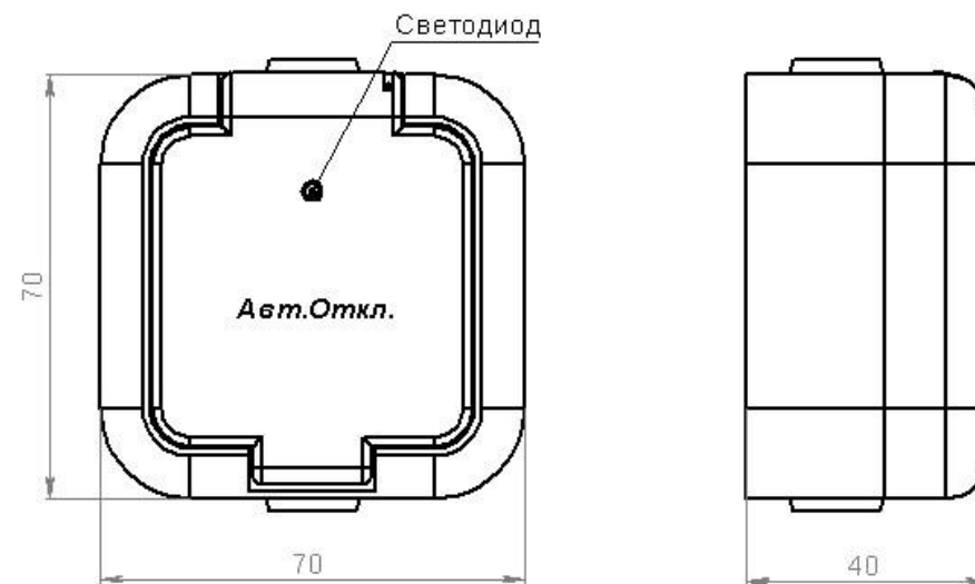
Рис. 2 Габаритные размеры считывателя.
