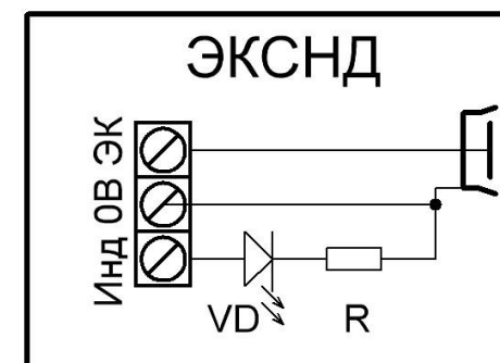
Рис.1 Схема подключения считывателя.
