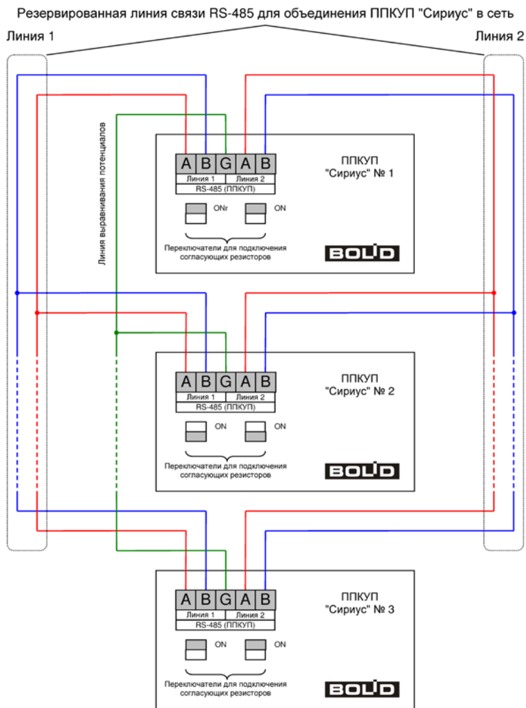
Рисунок 66. Схема объединения приборов «Сириус» в сеть
