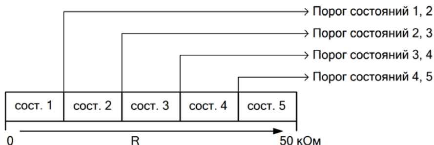
Рисунок 69. Состояния и пороги переходов между состояниями входа «Неисправность»
