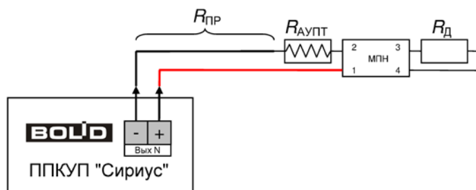
Рисунок 61. Рекомендуемая схема подключения АУПТ
