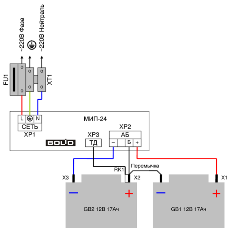
Рисунок 67. Схема подключения источников питания
