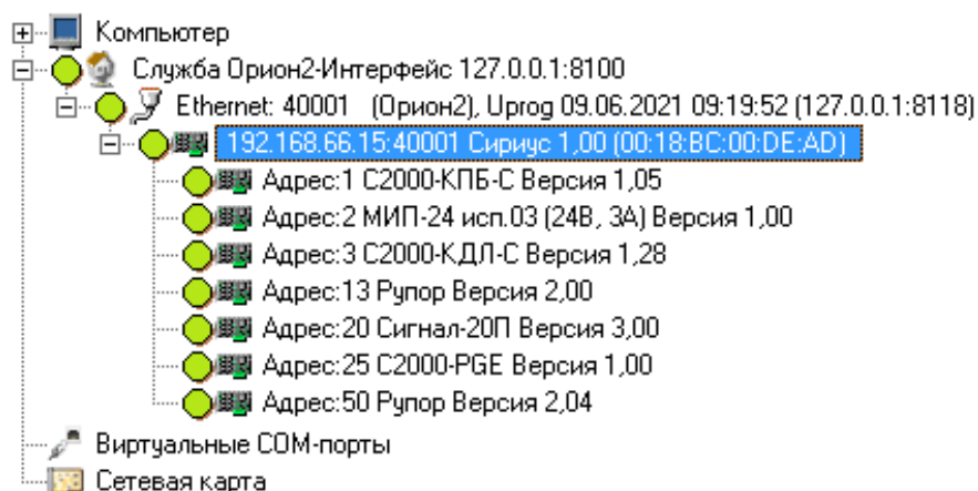
Рисунок 68. Дерево приборов в программе UProg
