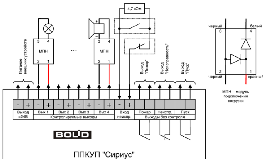
Рисунок 60. Схема подключения дискретных входов и выходов
