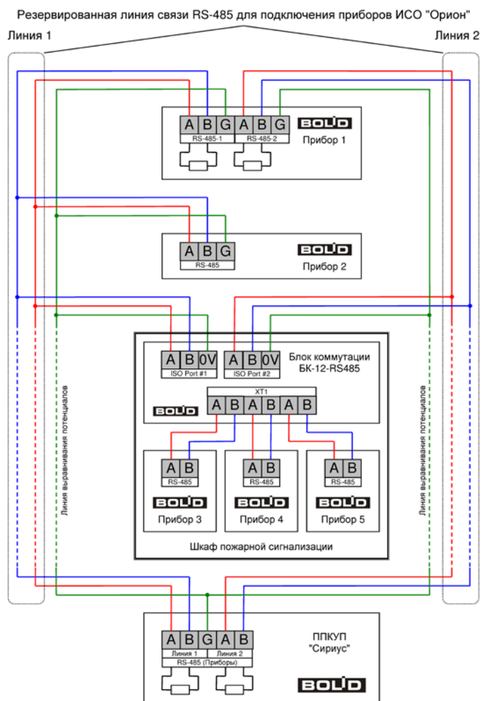
Рисунок 63. Схема подключения дополнительных блоков и приборов ИСО «Орион»
