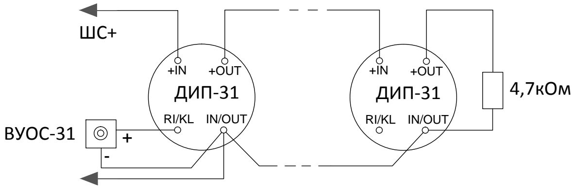
Схема подключения извещателей ИП435-8/101-04-А1R "СОНЕТ" в ШС типа 1 (сверху) и в ШС типа 2 (снизу)
